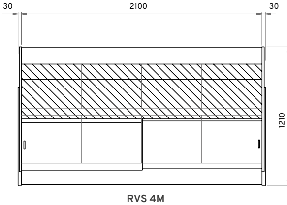
RVS 4M
