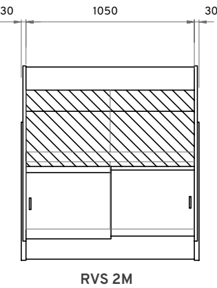
RVS 2M
