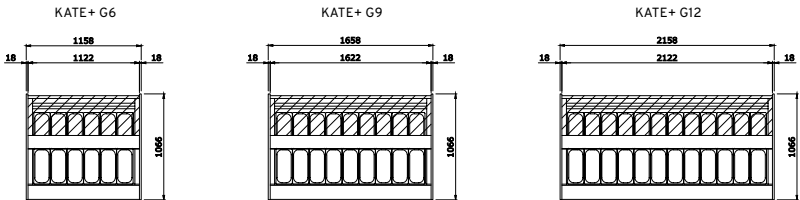
LATO OPERATORE VASCHE 360x165
