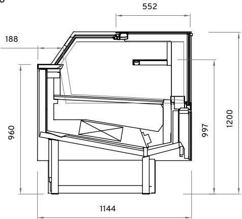
Sezione Section H 1200
